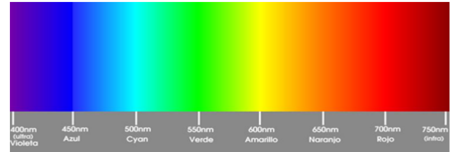
Espectro visible al ojo humano
